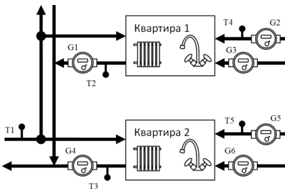
Рис.К.1 Учет тепла и воды в двух квартирах.
