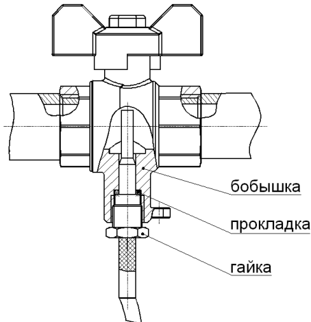
Рис. К.3 Монтаж термopреобразователя в корпусе шарового крана.
